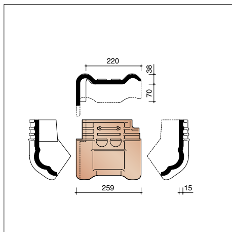
P9937280 Linker gevelknikpan
