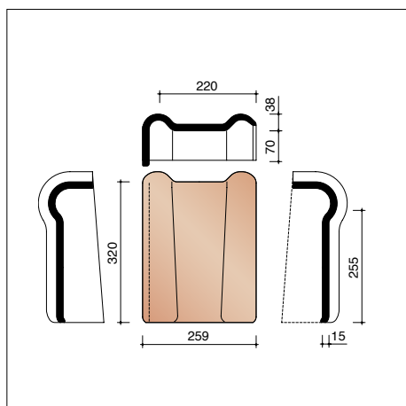
P9937580 Linker gevelhaakvorst
