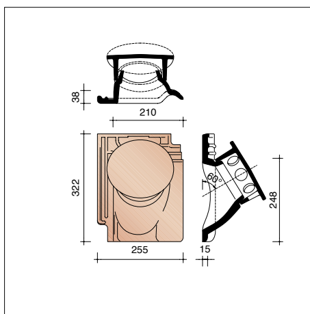
P9938741 Kit kokerpan Ø 100 mm + kapje - 95 cm 2 + aansluitingsmodule + reductorstuk
